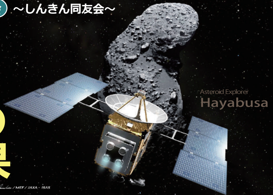
イトカワに接近する「はやぶさ」 © 池下章裕/MEF/JAXA・ISAS
